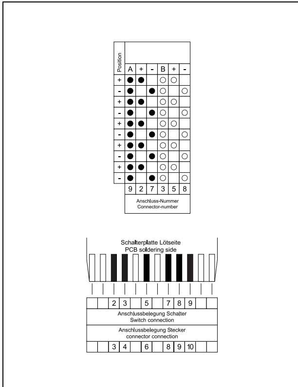
Code 011 Dezimal 0-10
