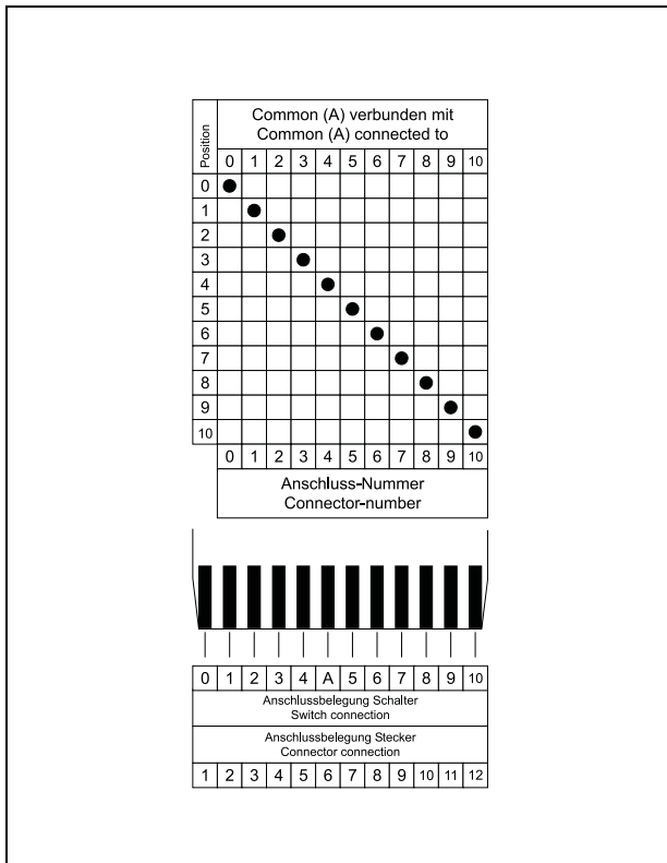
Code 011 Dezimal 0-10
