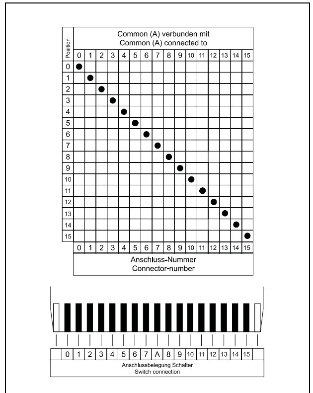
Code 016 Dezimal 0-15
